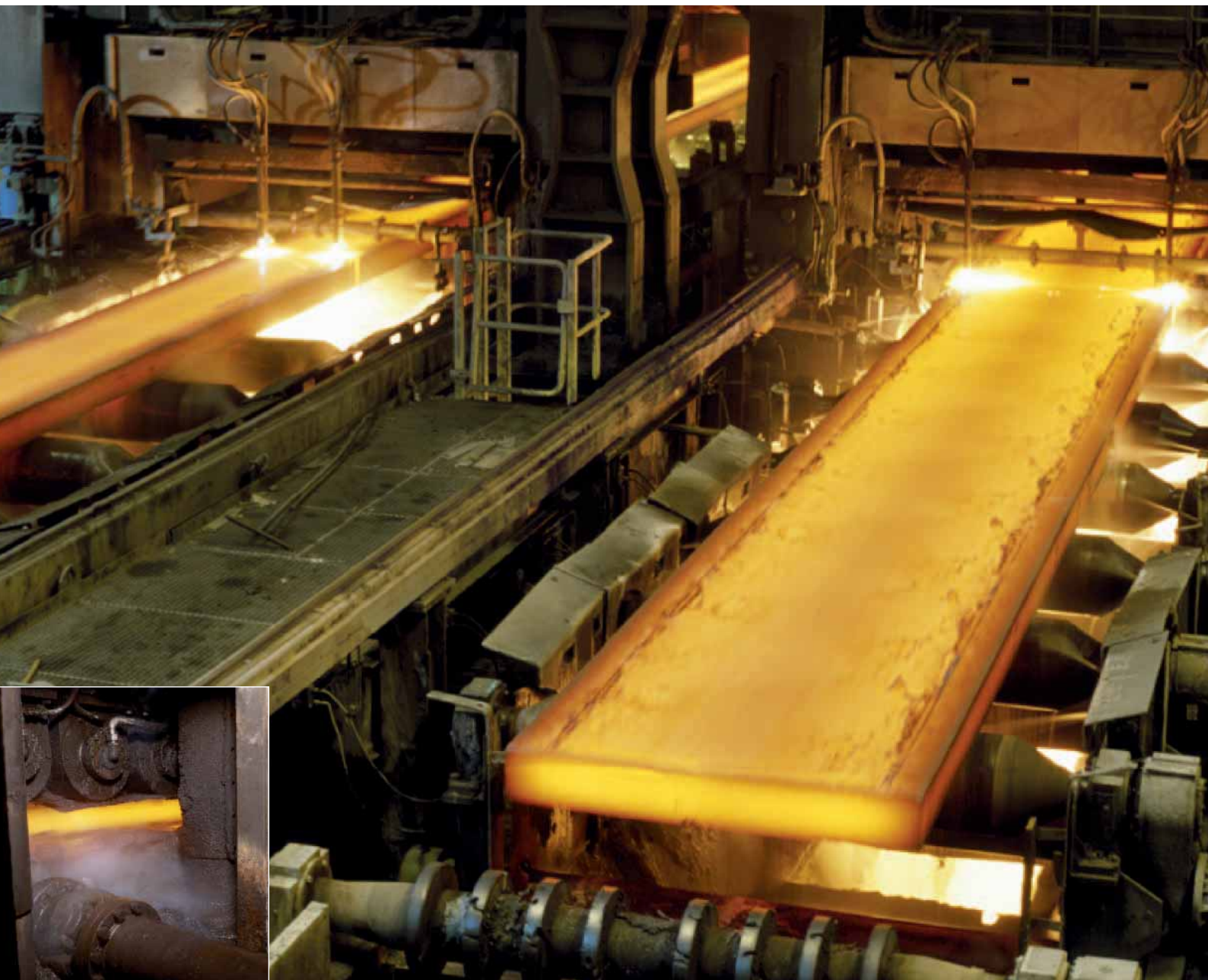
Ролики в МНЛЗ CGM 22
